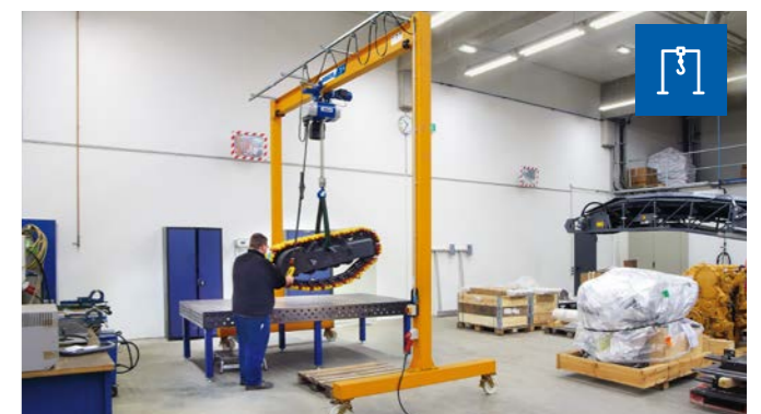
Handverrijdbare portaalkraan LPK
